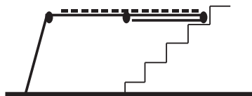
LEŠENÍ POUŽITÍ NA SCHODIŠTI (S PODLÁŽKOU)
